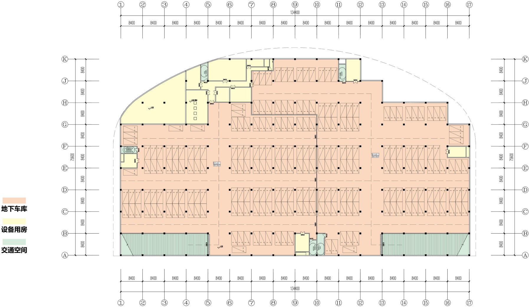
体育场下一层平面图
