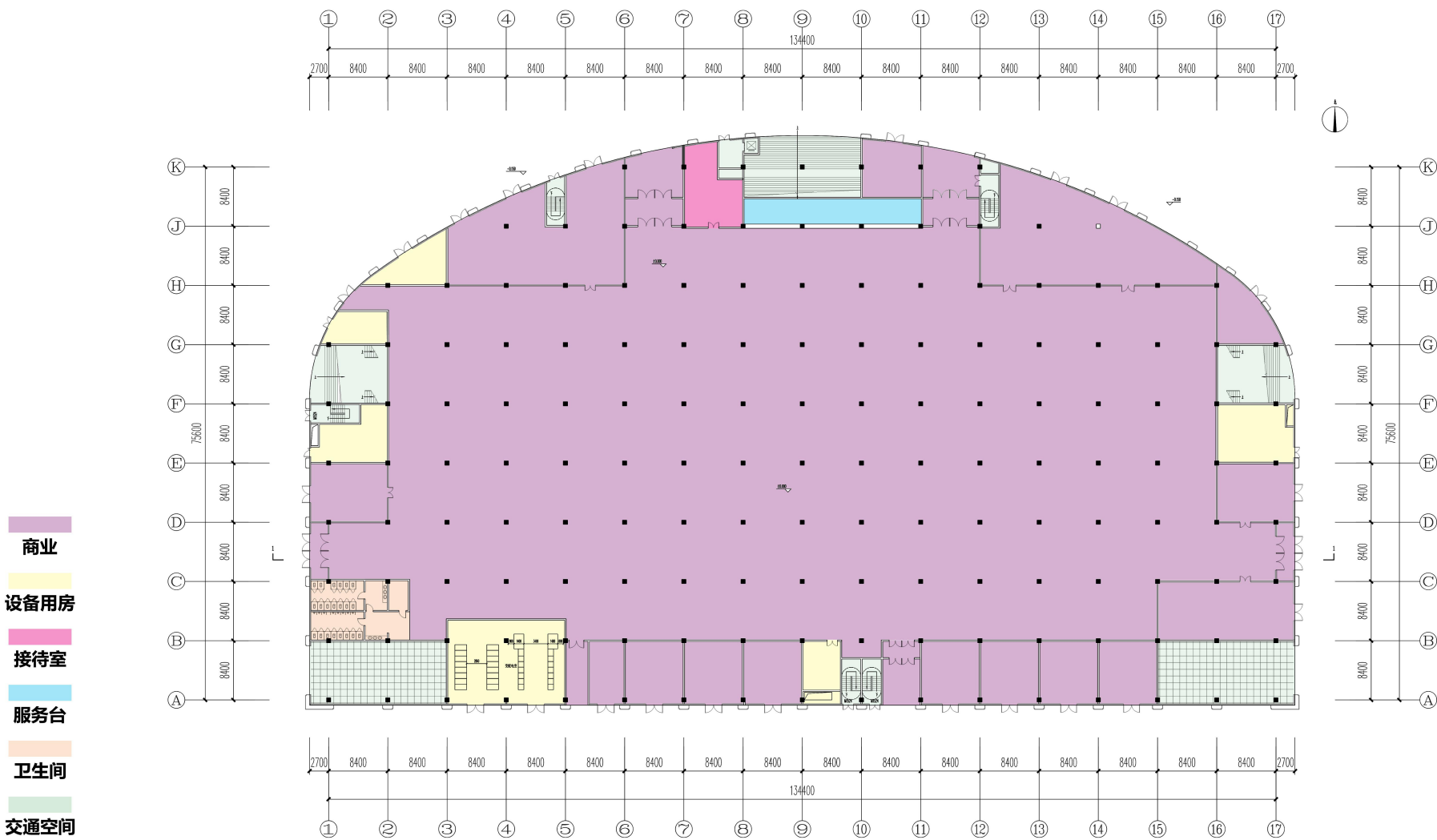
体育场一层平面图
