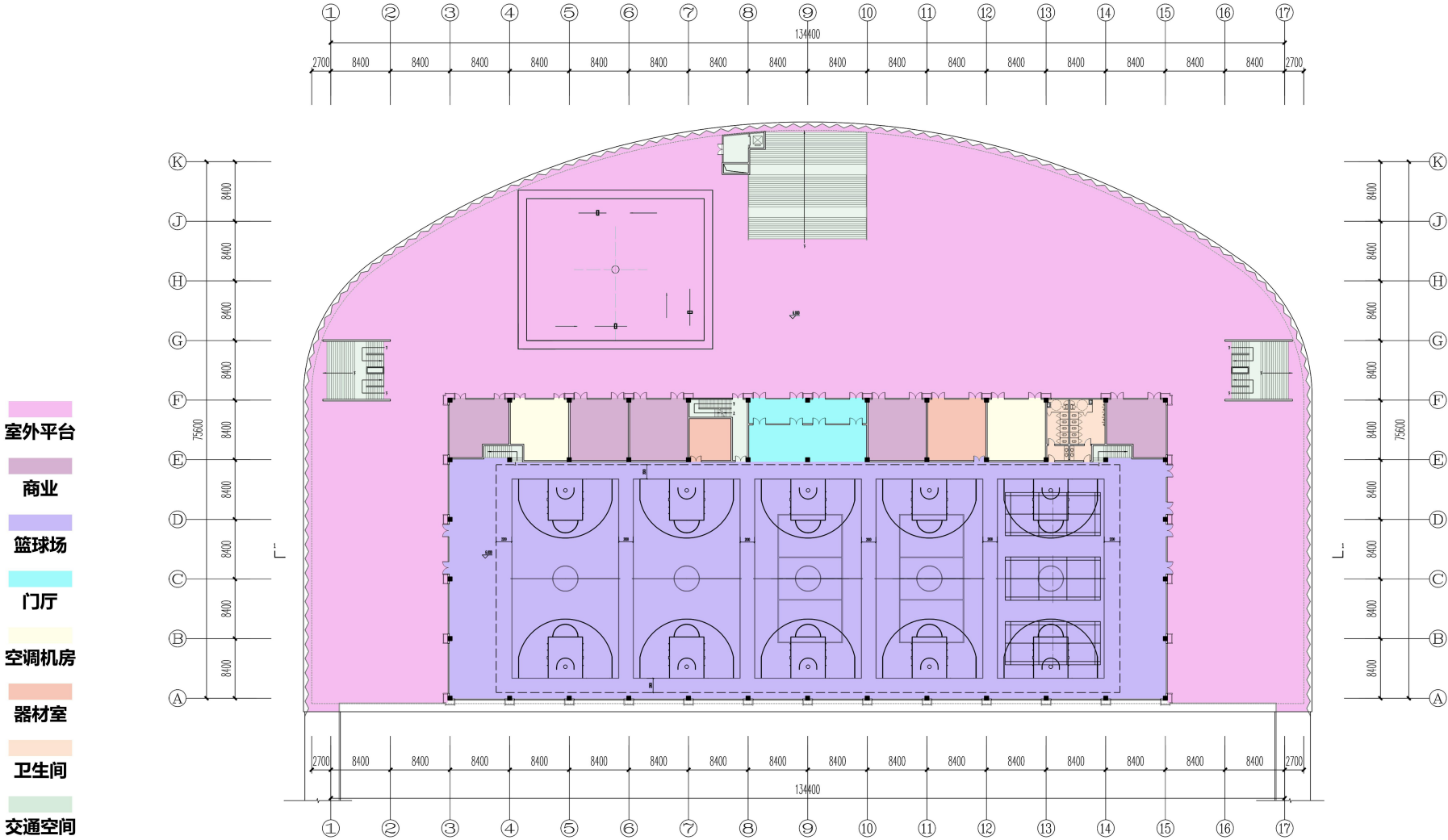
体育场二层平面图
